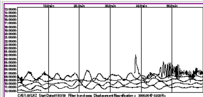
IU/CHTO, Chiang Mai, Thailand
