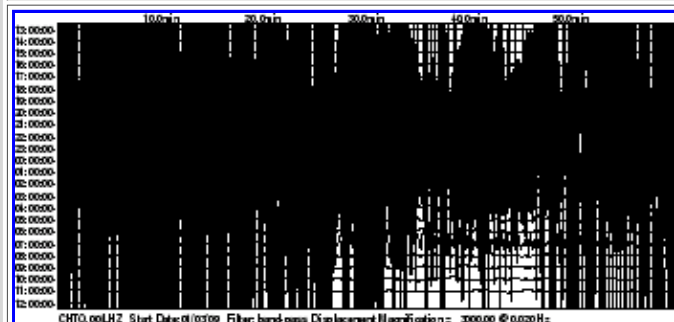
IU/COR, Corvallis, Oregon, USA
