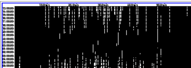
IU/TRIS, Tristan da Cunha, Atlantic Ocean
